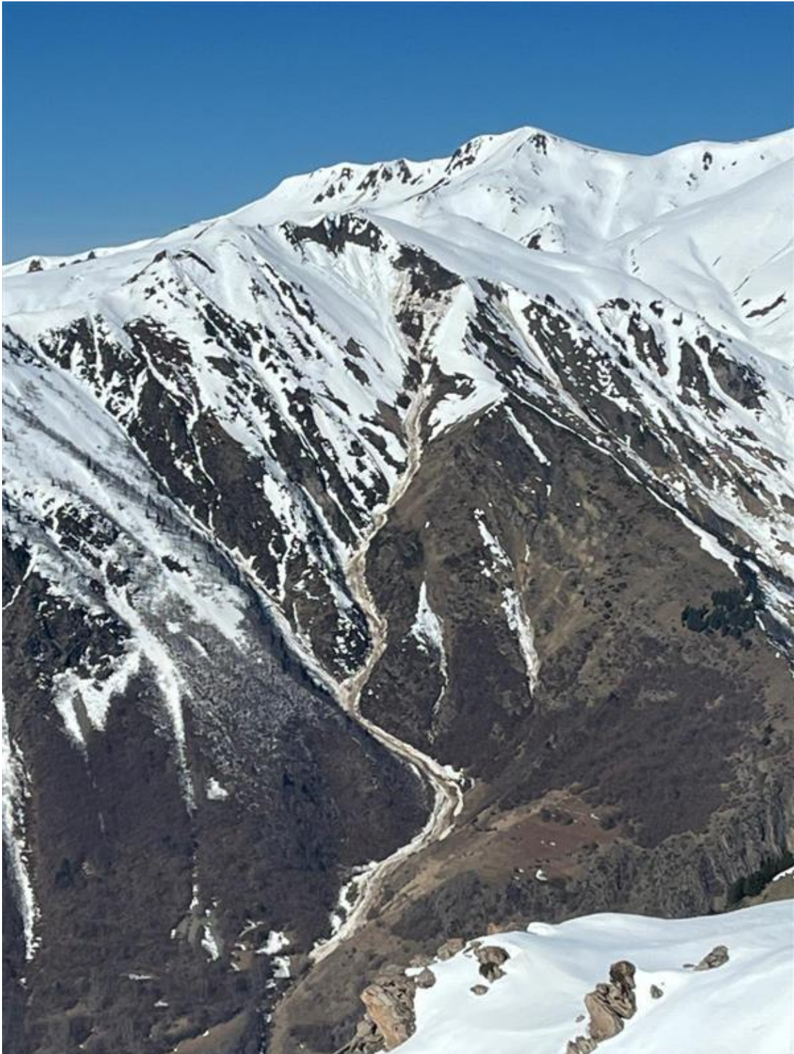
Lliscament basal de mida 3 (gran), observat dimecres 18 de març, a Baguerque (Aran).
