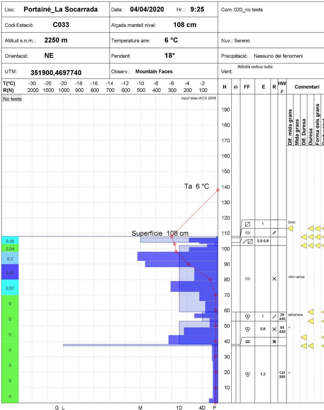
Perfil del dissabte 4 d'abril a Portainé-La Socarrada (Pallaresa), a 2250 m, en orientació nord-est. S'observa en superfície la neu recent en forma de partícules de precipitació fragmentades que s'estan facetant pel refredament superficial, damunt de crostes gruixudes que estableixen el conjunt del mantell.
