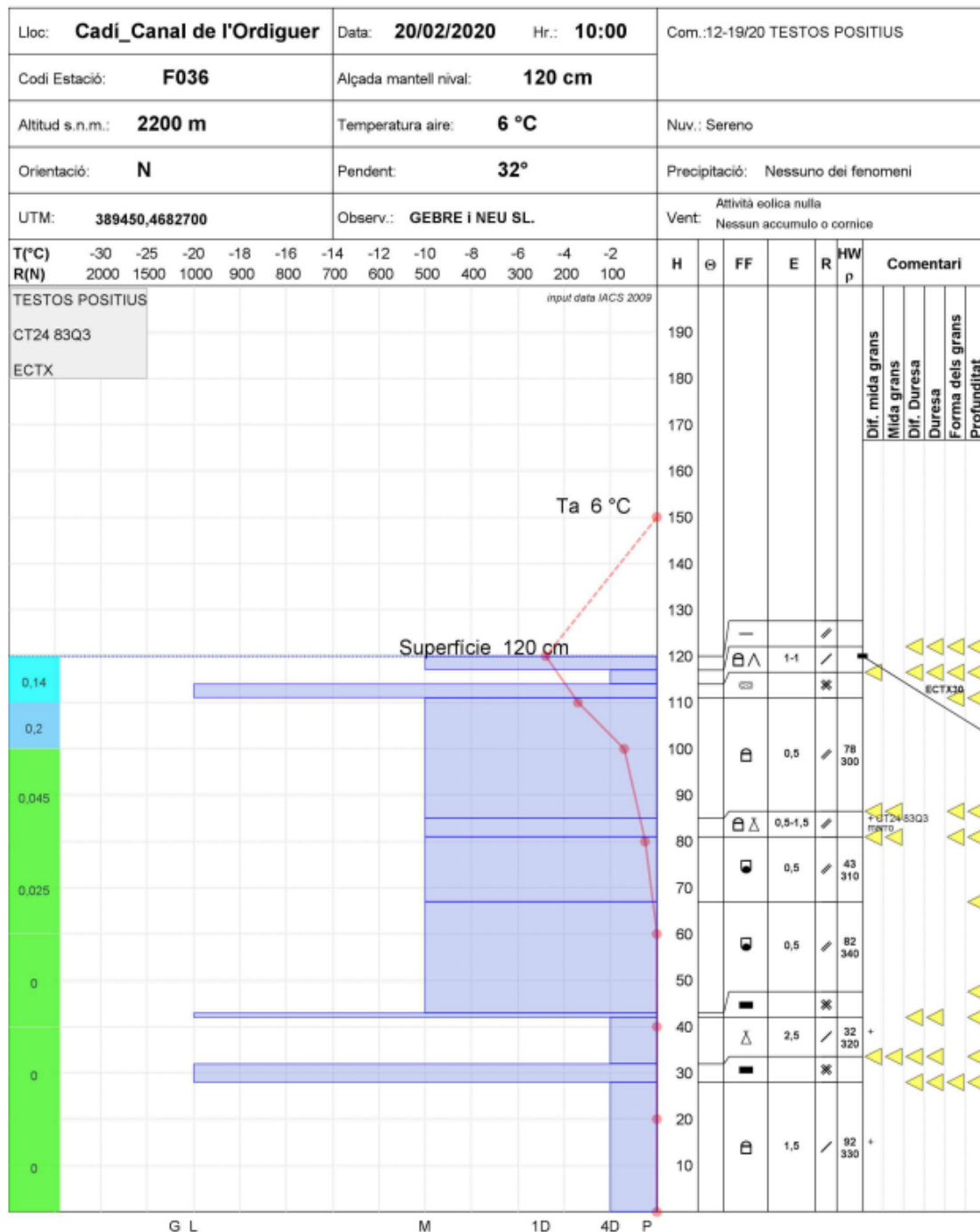
Perfil del mantell nival fet a la canal de l'Ordiguer (Vessant Nord Cadí-Moixeró) el 20 de febrer, en obaga a 2200 m. S'observen les capes febles persistents entre nivells encrostats. A destacar el refredament nocturn de la superfície del mantell.
